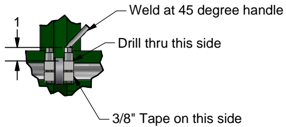
DETAIL B SCALE 0.14 : 1
